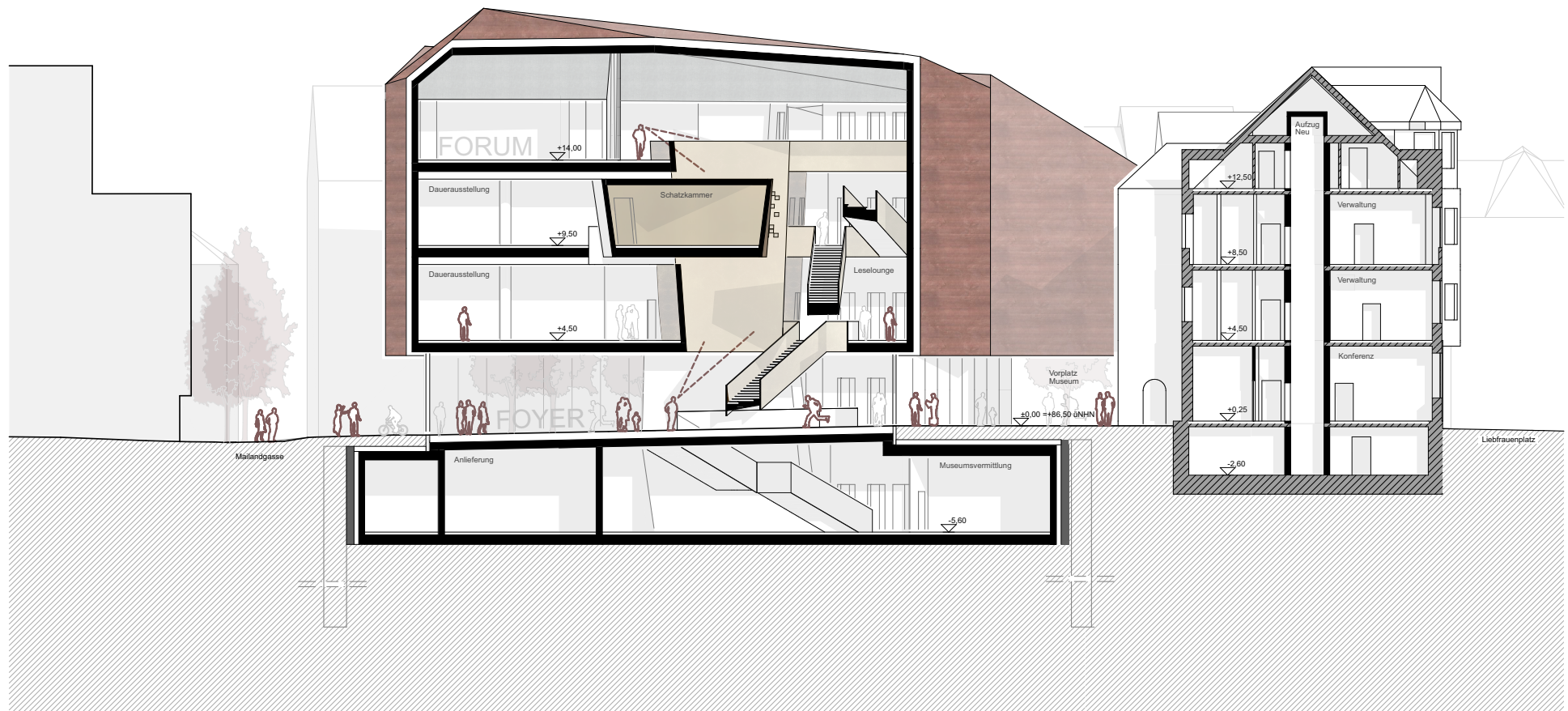
Arbeitsstand Querschnitt
